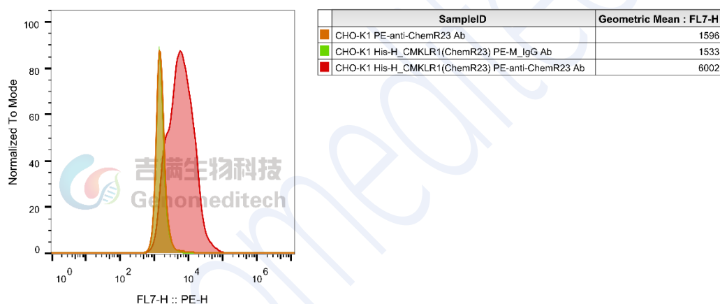
Fig 2.使用 Human ChemR23 PE-conjugated Antibody(R&D/FAB362P)抗体流式验证结果
