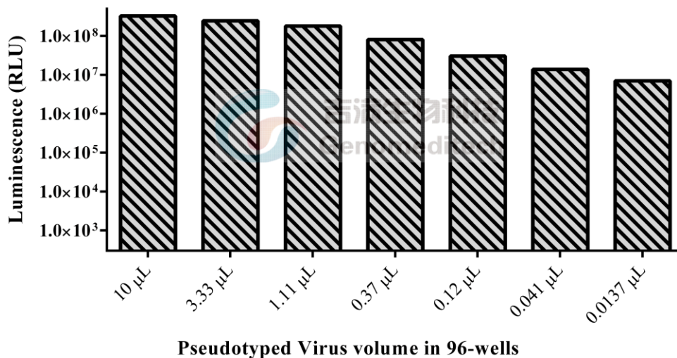
图2 吉满 SARS-CoV-2 Spike S 蛋白(BQ.1)突变型假病毒感染 HEK293T-ACE2 测定 Luciferase 数值
