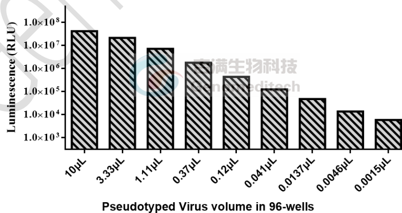
图 2 吉满 SARS-CoV-2 Spike S 蛋白(K417N+E484K+N501Y)突变型假病毒感染 HEK293T-ACE2 测定 Luciferase 数值
