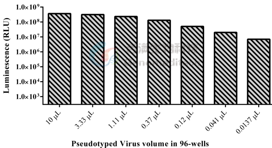
图2 吉满 SARS-CoV-2 Spike S 蛋白(XBB.1.9)突变型假病毒感染 HEK293T-ACE2 测定 Luciferase 数值
