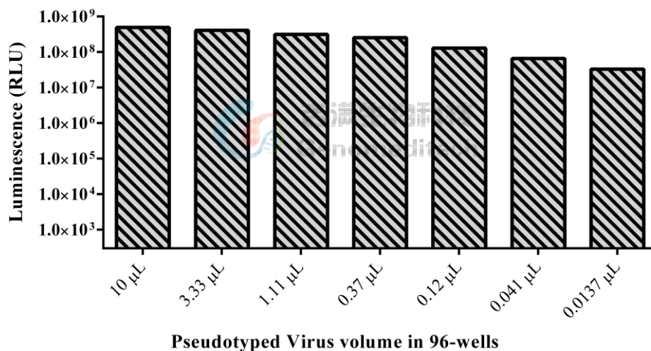
图2 吉满 SARS-CoV-2 Spike S 蛋白(EG.5.1)突变型假病毒感染 HEK293T-ACE2 测定 Luciferase 数值
