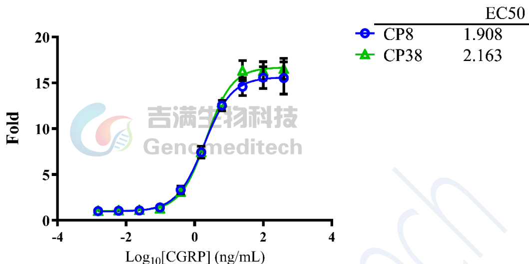
Fig 4. 制备 CGRP (Human) (phoenixpeptide/015-02) 梯度稀释液; 提前 16-24 h 配置 H_CALCRL RAMP1 Reporter HEK-293 DDX35 TM Cell Line (Genomeditech/GM-C37743), 每孔细胞量 1.5 \times 10^4 个。将过夜培养的细胞吸弃上清, 加入稀释好的 CGRP (Human), 3 复孔, 孵育 7 h 后检测 Luciferase 数值, 使用 GraphPad 系统进行数据分析, 纵坐标转换为倍率。结果显示, CP8 代与 CP38 代倍率、EC50 数值稳定。
