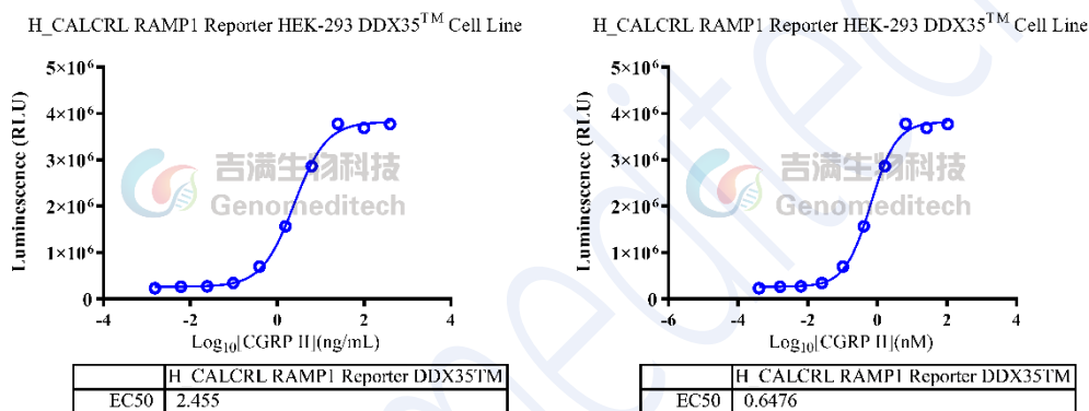
Fig 7. CGRP II 药物验证结果（右图对药物进行质量浓度和摩尔浓度的换算后绘制）
