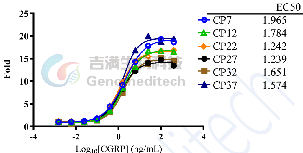
Fig 2. 制备 CGRP (Human) (phoenixpeptide/015-02) 梯度稀释液；提前 16-24 h 配置 H_CALCRL RAMP1 Reporter HEK-293 DDX35 TM Cell Line (Genomeditech/GM-C37743)，每孔细胞量 1.5 \times 10^4 个。将过夜培养的细胞吸弃上清，加入稀释好的 CGRP，孵育 7 h 后检测 Luciferase 数值，使用 GraphPad 系统进行数据分析，纵坐标转换为倍率。结果显示，不同代次间倍率、EC50 数值稳定。
