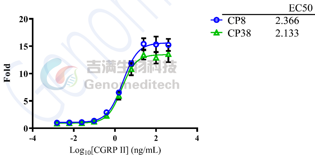
Fig 5. 制备 CGRP II (Human) (phoenixpeptide/015-07) 梯度稀释液; 提前 16-24 h 配置 H_CALCRL RAMP1 Reporter HEK-293 DDX35 TM Cell Line (Genomeditech/GM-C37743), 每孔细胞量 1.5 \times 10^4 个。将过夜培养的细胞吸弃上清, 加入稀释好的 CGRP II, 3 复孔, 孵育 7 h 后检测 Luciferase 数值, 使用 GraphPad 系统进行数据分析, 纵坐标转换为倍率。结果显示, CP8 代与 CP38 代倍率、EC50 数值稳定。
