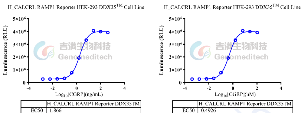
Fig 6. CGRP 药物验证结果（右图对药物进行质量浓度和摩尔浓度的换算后绘制）
