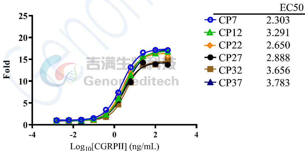
Fig 3. 制备 CGRP II (Human) (phoenixpeptide/015-07) 梯度稀释液；提前 16-24 h 配置 H_CALCRL RAMP1 Reporter HEK-293 DDX35 TM Cell Line (Genomeditech/GM-C37743)，每孔细胞量 1.5 \times 10^4 个。将过夜培养的细胞吸弃上清，加入稀释好的 CGRP II，孵育 7 h 后检测 Luciferase 数值，使用 GraphPad 系统进行数据分析，纵坐标转换为倍率。结果显示，不同代次间倍率、EC50 数值稳定。
