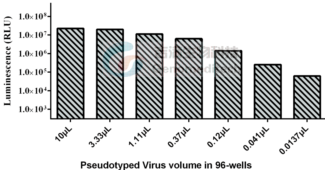
图2 吉满 SARS-CoV-2 Spike S 蛋白(D614G+I472V)突变型假病毒感染 HEK293T-ACE2 测定 Luciferase 数值
